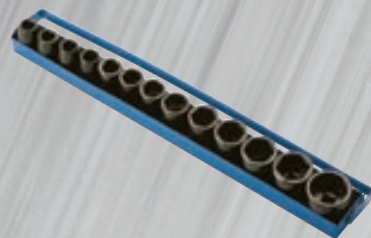
SERIE BUSSOLE AD IMPATTO, SERIE NORMALE
