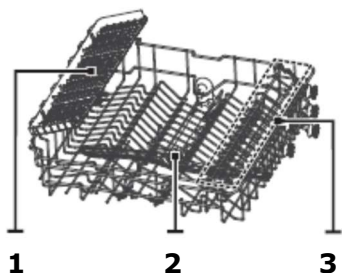
Горна кошница: 1) Поставка за прибори 2) Горно разпръскващо рамо 3) Поставка за чаши
