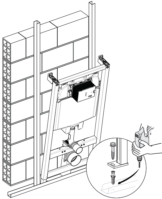
Sistema con rivestimento a secco Dry wall system
