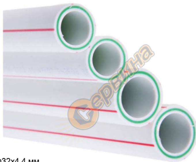
Ф32x4.4 мм PN20
